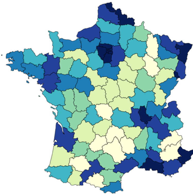
Figure 73. Choropleth (Gregor Aisch)
